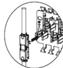
Posizionamento giunto Coupler positioning
