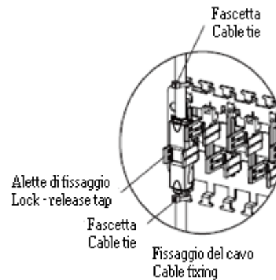
Posizionamento giunto Coupler positioning
